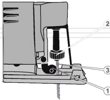
Рисунок 2. Схема встановлення та вилучення ріжучого полотна.
