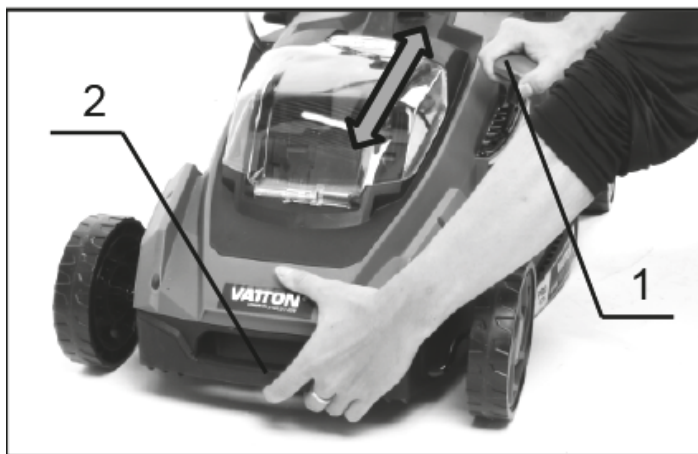
Рисунок 9. Схема регулювання висоти скошування.
