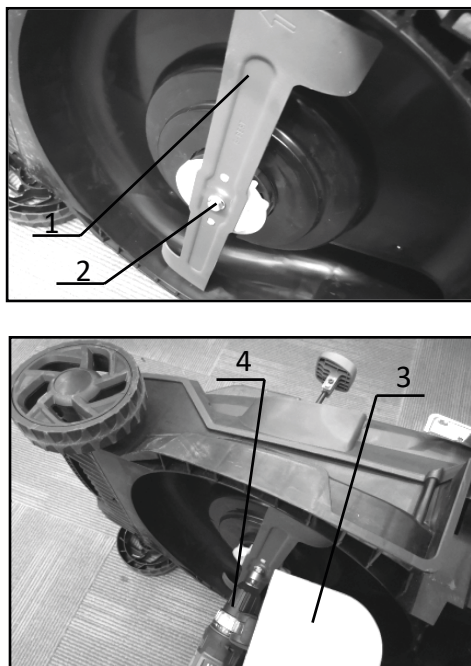
Рисунок 14. Схема демонтажу ножа.
