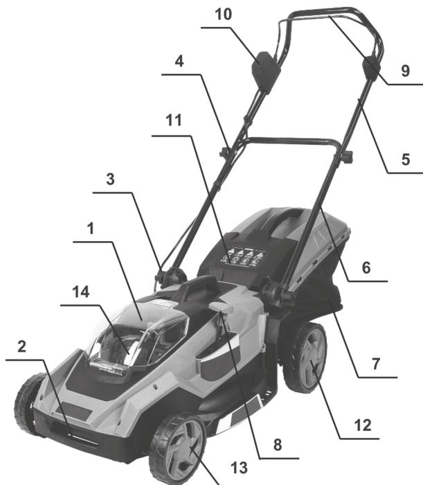
Рисунок 1. Загальний вигляд виробу.
