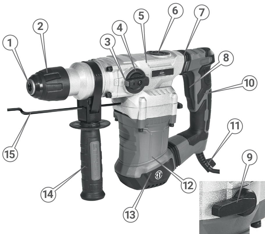
Рисунок 1. Загальний вигляд перфоратора.
