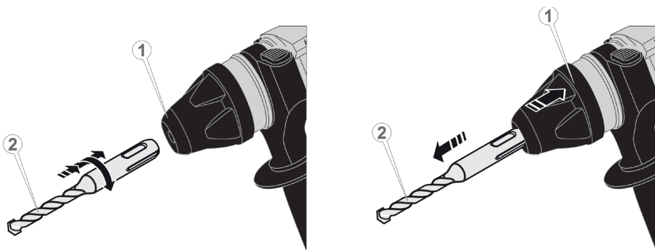
Рисунок 4. Схема встановлення/вилучення змінного кінцевого інструмента.
