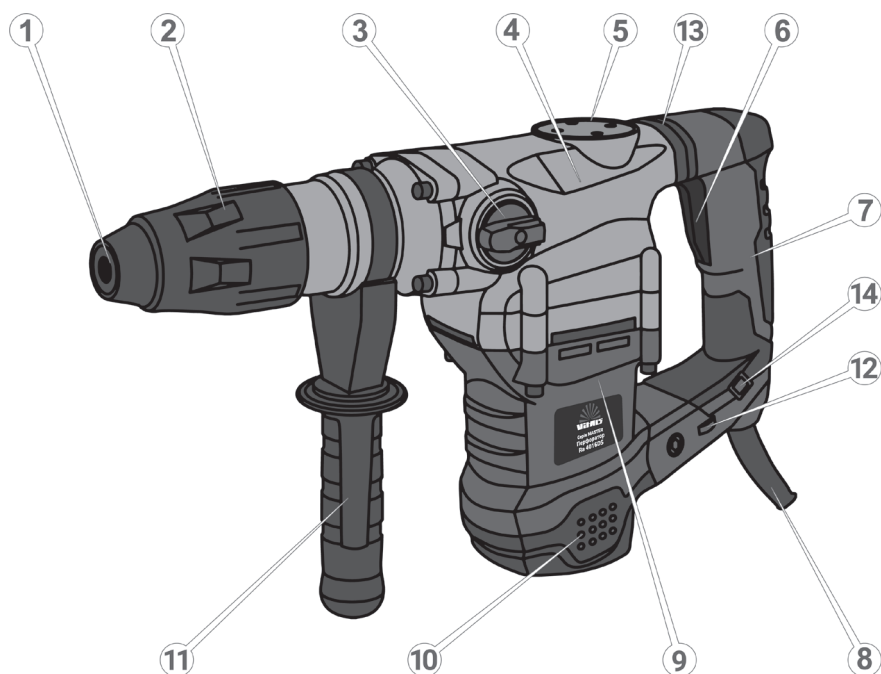
Рисунок 1. Загальний вигляд перфоратора електричного.
