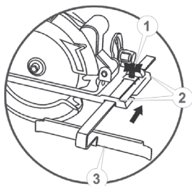
Рисунок 6. Схема встановлення паралельної напрямної.
