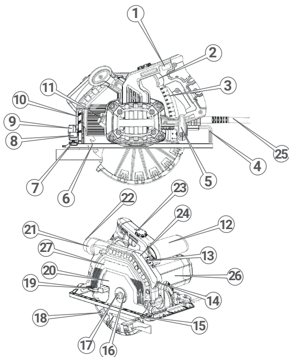
Рисунок 1. Загальний вигляд виробу.
