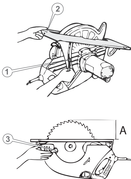
Рисунок 4. Схема регулювання глибини різь.
