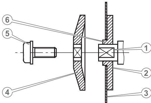
Рисунок 2. Схема встановлення циркулярного диска.
