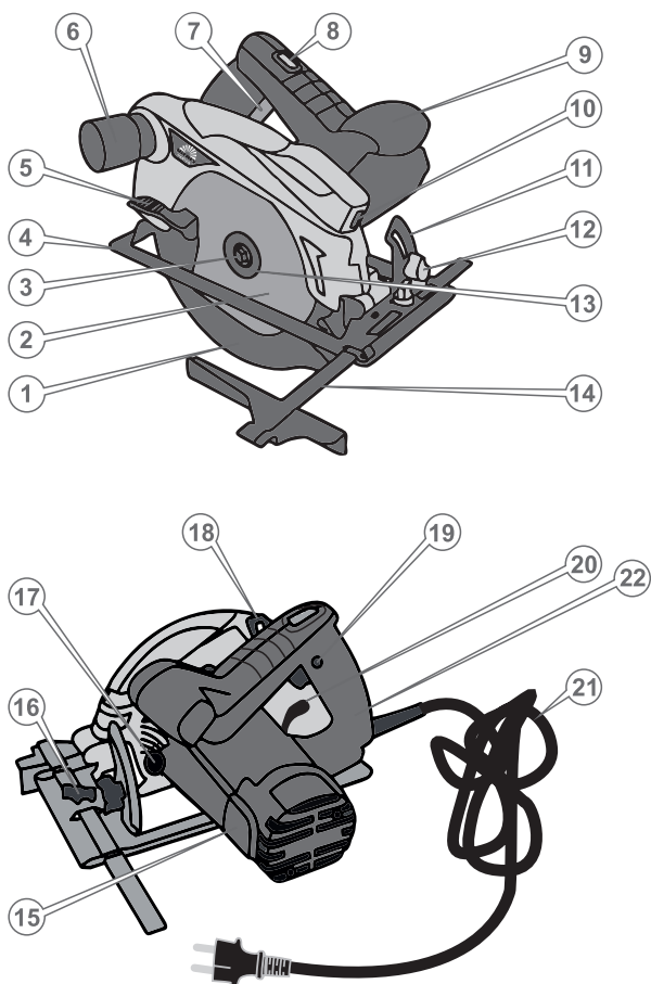
Рисунок 1. Загальний вигляд циркулярної пили Vitals Master, модель «Rg 1912XCla»
