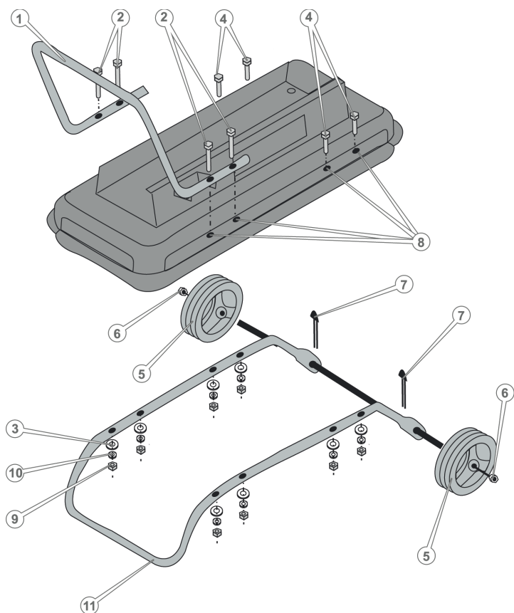
Рисунок 2. Схема складання виробу.
