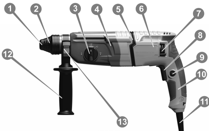
Рисунок 1. Загальний вигляд перфоратора. Модель «Ra 2811NCv».
